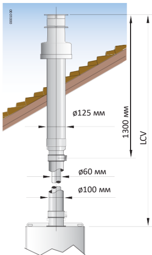
Пример вертикальной коаксиальной системы.
