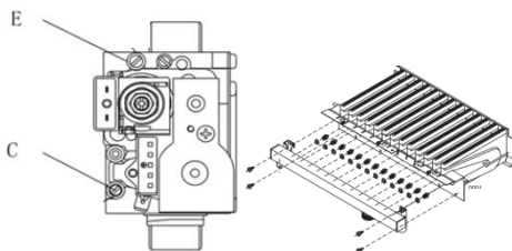
Газовая арматура PIONEER PLUS F
